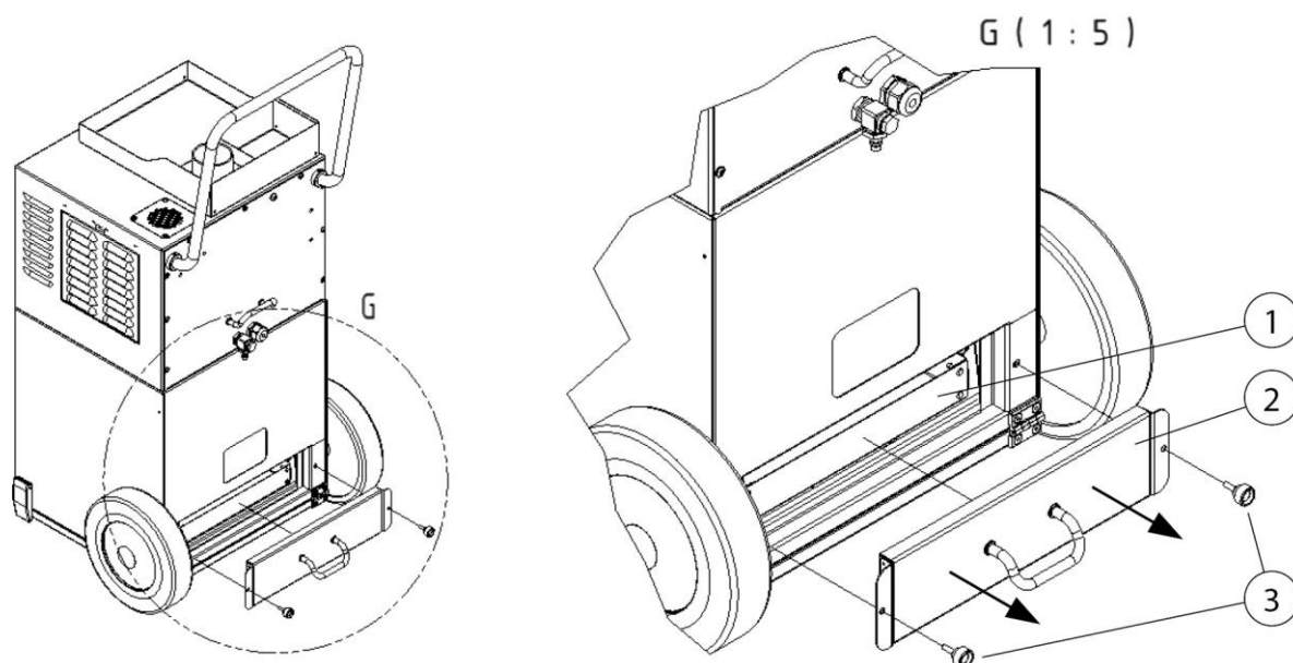
Fig. 6: Sostituzione del collettore di polvere
