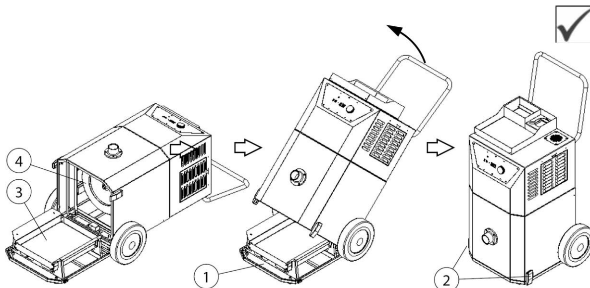
Fig. 13: chiudere il coperchio di manutenzione
