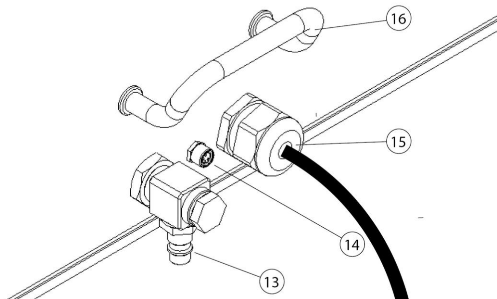
Fig. 2: Collegamenti
