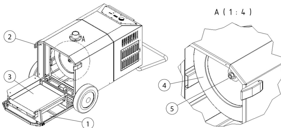
Fig. 10: Cambio del filtro
